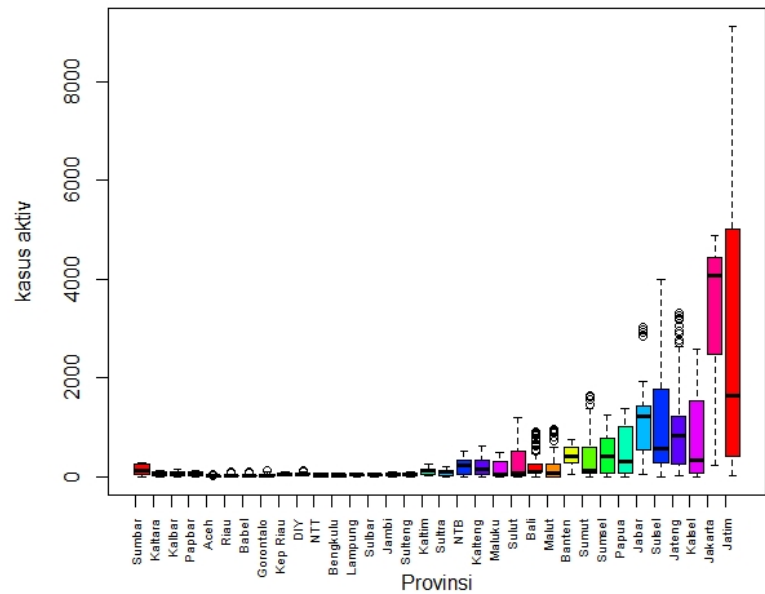
Gambar 3. Boxplot Kasus Aktiv COVID-19 Per-Provinsi di Indonesia
