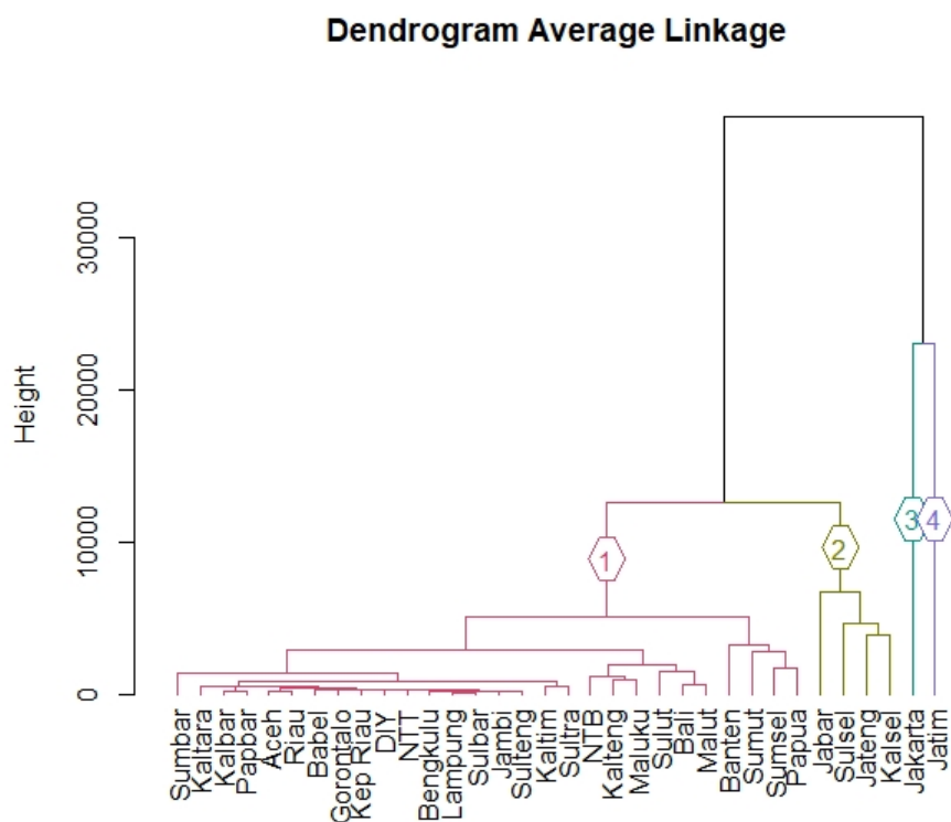
Gambar 4. Dendrogram Hasil Pengelompokkan berdasarkan Algoritma Average Linkage
