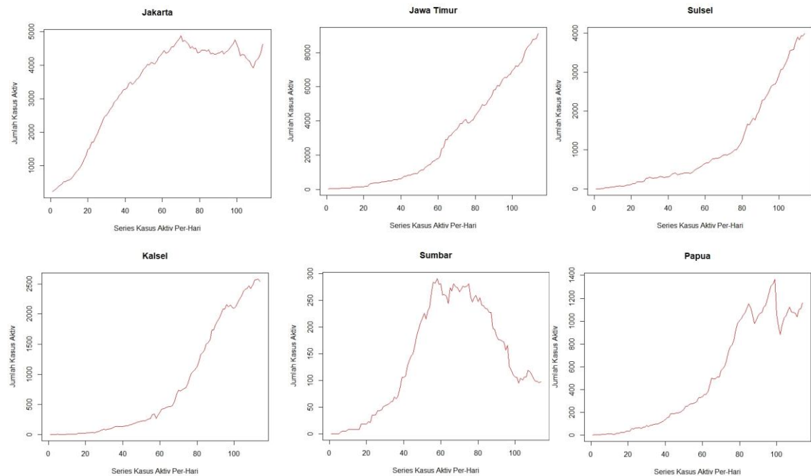
Gambar 1. Grafik Deret Waktu Kasus Aktif COVID-19
