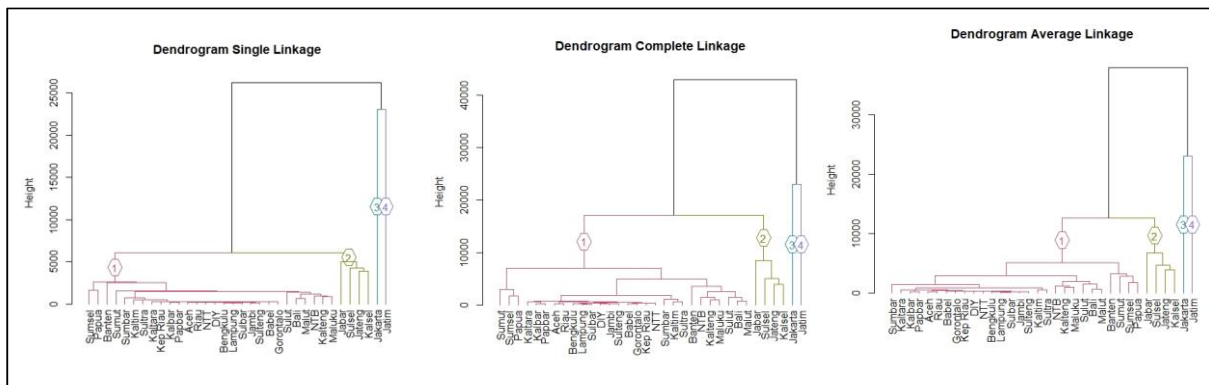
Gambar 2. Dendrogram Hasil Pengelompokan berdasarkan Algoritma Single , Complete dan Average Linkage
